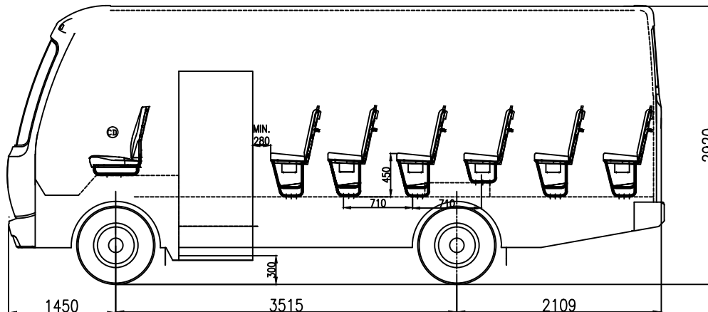
LH SIDE
